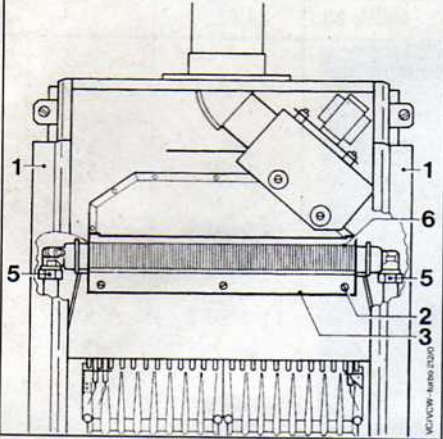
Afb. 14 1 Zijwanden 2 Schroeven 3 Afdekplaat 5 Koppeling 6 Warmtewisselaar
